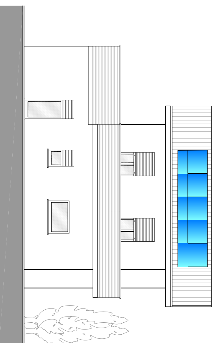
PROSPETTO OVEST
