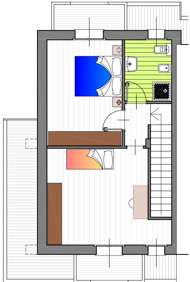
PIANTA PIANO PRIMO bifamiliare porzione C 1
