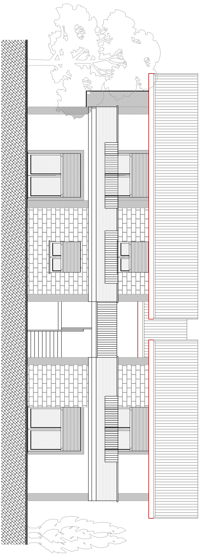
PROSPETTO SUD
